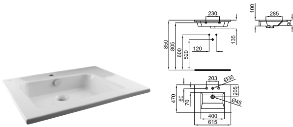
80 cm. wall hung basin with overflow and fixing kit 100041225 - N421040000. Lavabo 60 cm. suspendu avec trop plein et fixations 100041225 - N421040000.
