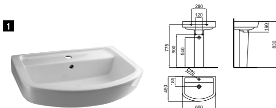
1 60 cm. wall hung basin with overflow and fixing kit 100041225 - N421040000. Lavabo 60 cm. avec trop plein et fixations 100041225 - N421040000.
