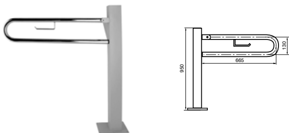
Vertical double folding grab rail with floor support and roll holder Barre de maintien double verticale avec pied et porte-papier
