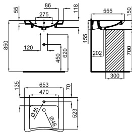
1 65cm wall hung basin, with overflow. Includes the fixings kit 100041225 - N421040000 Lavabo 65 cm. suspendu avec trop plein et fixations 100041225 - N421040000. Spécial pour PMR
