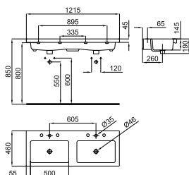
1 120 cm. wall hung basin with fixing kit 100041225 - N421040000 with overflow. Lavabo 120 cm. suspendu à bac double avec trop plein et fixations 100041225 - N421040000.
