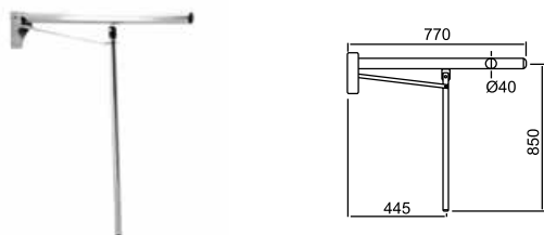
Vertical folding rail Barre rabattable verticale pour mur plâtre
