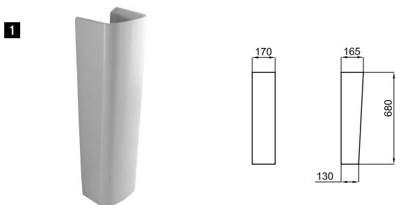
1 Pedestal for basin 60 cm. and cloakroom basin 50 cm. . Colonne pour lavabo 60 cm. et lave-mains 50 cm .
