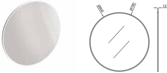
1 LOUNGE. Ø80 cm Mirror with lacquered wood frame Miroir Ø80 cm avec cadre en bois laqué
