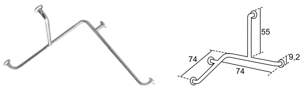
1 70x74 cm. corner grab rail Barre horizontale d'angle 70x74 cm.
