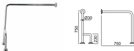
Grab rail 3 wall-floor Barre de maintien fixation sol-mur
