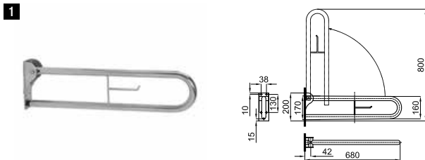
1 68 cm vertical folding grab rail with roll holder Barre de maintien rabattable verticale 68 cm. avec porte-papier
