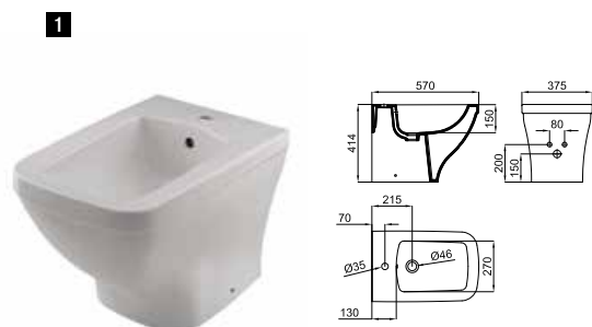
1 Bidet with fixing kit 100110005 - N499816959 Bidet avec fixations 100110005 - N499816959
