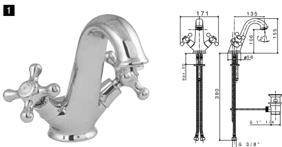
1 Monoblock basin mixer 3/8". ceramic disc valves . Length of hoses 390 mm. with pop-up waste set 1 1/4". "Plus" aerator. Flow rate 17,69 l/min. at 3 bar. Mélangeur lavabo tête céramique . Flexibles raccordement 3/8" longueur 390 mm., garniture de vidage 1 1/4". Avec mousseur "plus". À 3 bars de pression 17,69 l/min.
