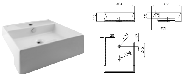
AZOR. 47x46 cm. semi-recessed basin with overflow. Lavabo 47x46 cm. à encastrer avec trop plein.
