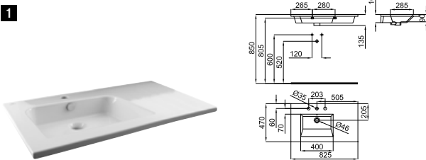
1 80 cm. wall hung basin with overflow and fixing kit 100041225 - N421040000. Lavabo 80 cm. suspendu avec trop plein et fixations 100041225 - N421040000.
