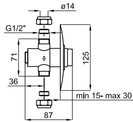
Concealed flush valve 1/2" for urinals. Fluxomètre poussoir encastré pour urinoir. Installation : encastré mur solide.
