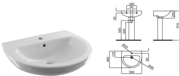
56 cm. wall hung basin with overflow and fixing kit 100041151 - N401150000. Lavabo 56 cm. avec trop plein et fixations 100041151 - N401150000.
