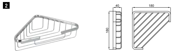
2 Corner soap basket Porte-savon d'angle
