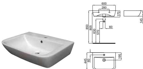
60 cm. wall hung basin with overflow and fixing kit 100041225 - N421040000 Lavabo 60 cm. avec trop plein et fixations 100041225 - N421040000
