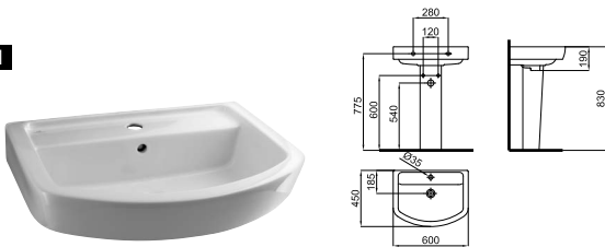
1 ACRO. 60 cm. wall hung basin with overflow and fixing kit 100041225 - N421040000. Lavabo 60 cm. avec trop plein et fixations 100041225 - N421040000.
