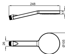
1 HOTELS - Single position handshower with AIR ECO system . Flow rate 12 l/min. at 3 bar. HOTELS - Douchette 1 position avec système AIR ECO . À 3 bars de pression 12 l/min.
