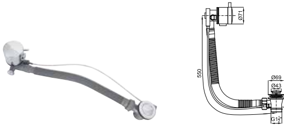
Overflow bath filler Trop-plein avec robinet baignoire
